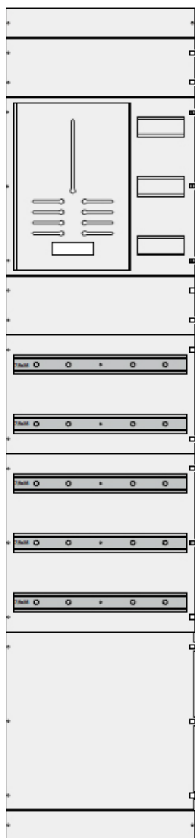
■ INNREDNING 450MM ■ VARENUMMER 990254
