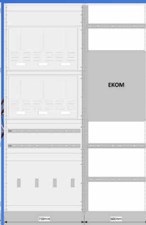
BESTILLINGSNUMMER 990023 ETASJEFORDELER 6 MÅLERE MED NH LASTBRYTER/NM8 EFFEKTBRYTER
